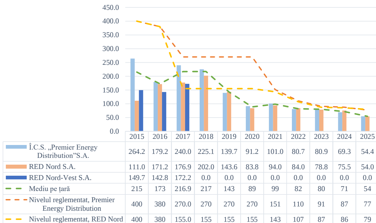
Figura 19. Evoluția indicatorului SAIDI, min. (2015-2025) Sursa: ANRE
